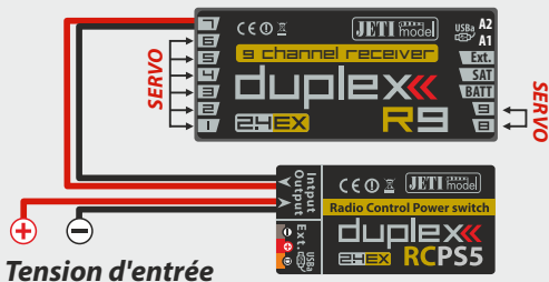
Fig. 5: Exemple de connexion avec RC Power Switch
